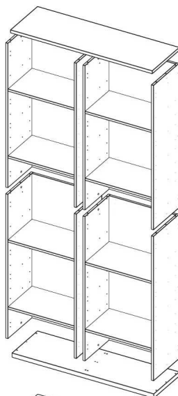
Korkeus 225 cm Modulit: Runko korkea 4 kpl
