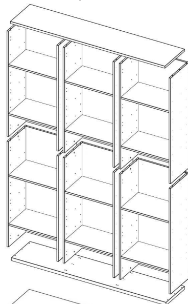
Leveys 162 cm Moduli: Kansi + pohja 162 cm
